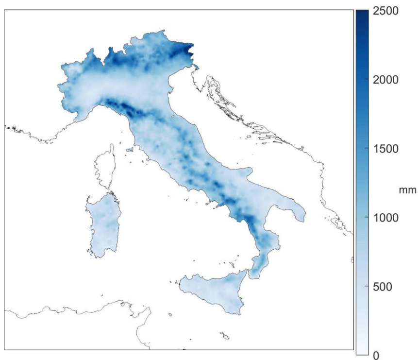
Figura 5.1: Precipitazione cumulata 2023.
