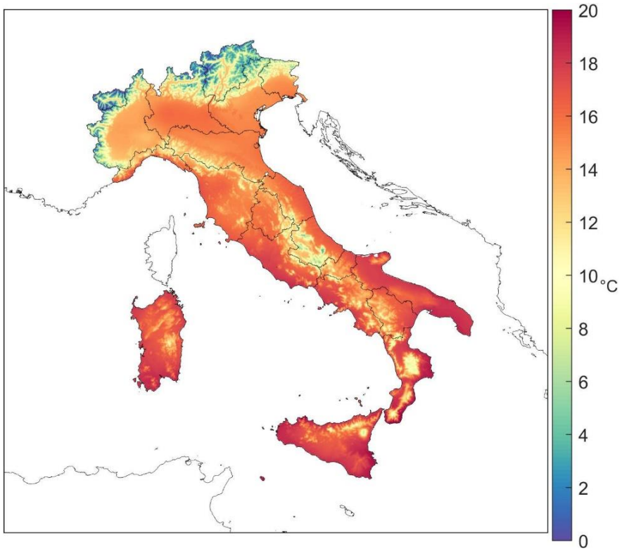
Figura 3.1: Temperatura media 2023.
